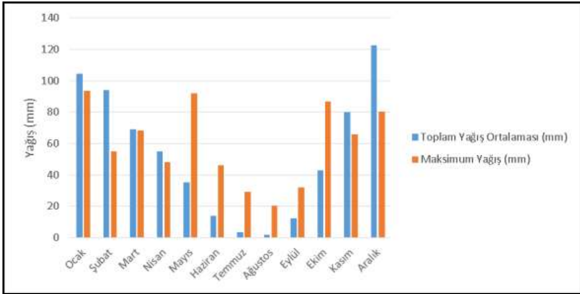
Şekil 19. Aydın Meteoroloji İstasyonu Verilerine Ait Yağış Değerleri Grafiği
