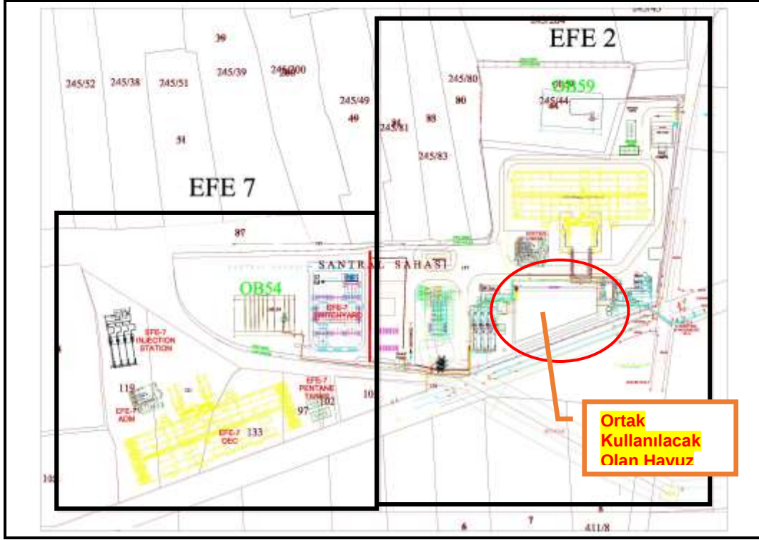
Şekil 12. Vaziyet Planı ve Planlanan Ortak Kullanım
