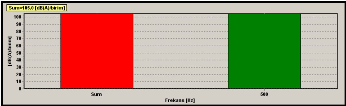
Şekil 101. Paletli Vince Ait Gürültü Düzeyinin Frekans Analizi
