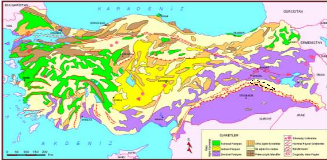
Şekil 39. Türkiye'nin Genel Tektonik Haritası
