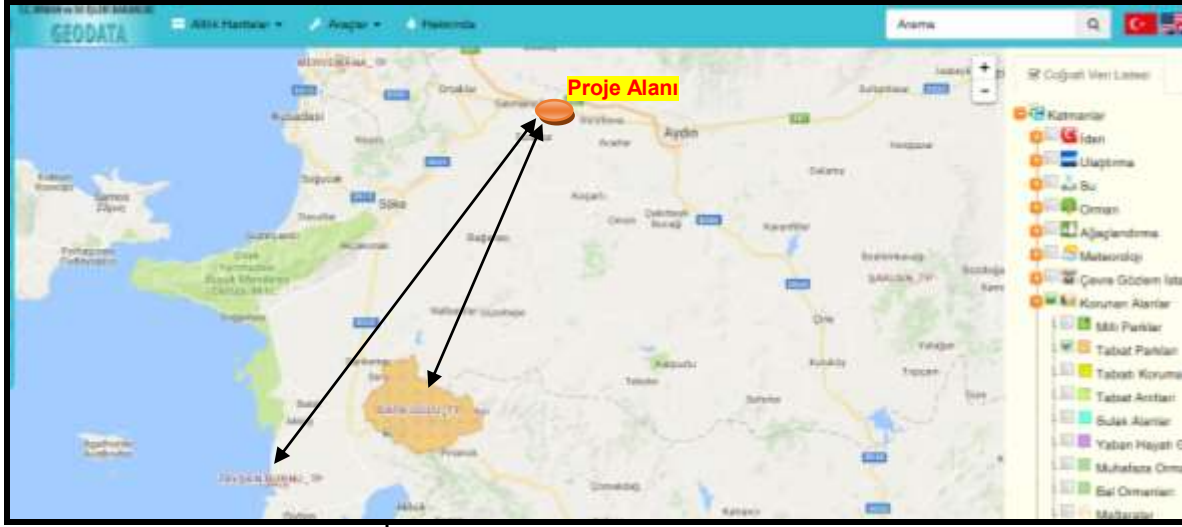
Şekil 64. Proje Alanı ve Aydın İli Sınırlarındaki Tabiat Parklarını Gösterir Harita-1
