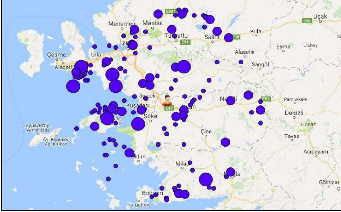
Şekil 43. Proje Alanının Yer Aldığı 100 km Çaplı Alandaki Büyük Depremler
