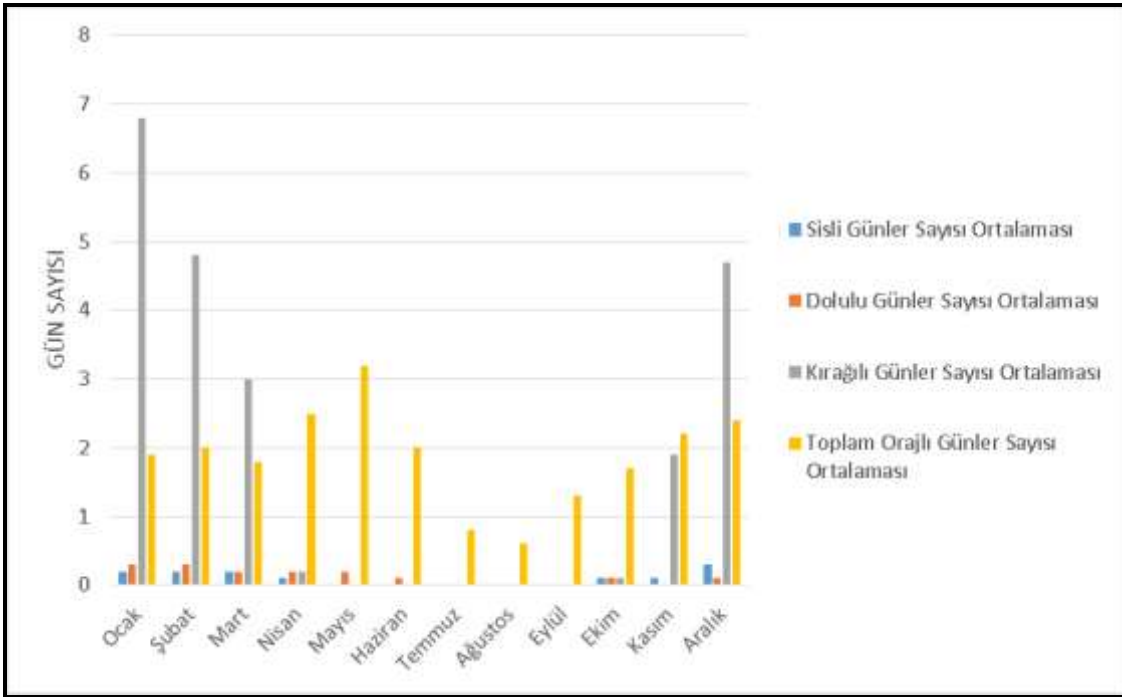
Şekil 22. Aydın Meteoroloji İstasyonuna Ait Sisli, Dolulu, Kırğılı ve Toplam Orajlı Gün Sayıları Grafiği
