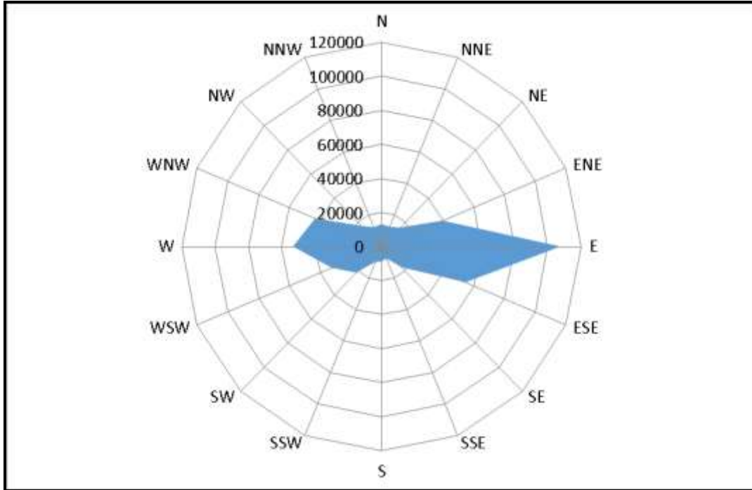
Şekil 28. Aydın Meteoroloji İstasyonuna Ait Rüzgarın Esme Sayılarına Göre Yıllık Rüzgar Diyagramı
