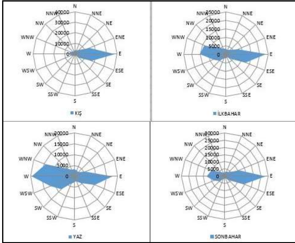
Şekil 30. Aydın Meteoroloji İstasyonuna Ait Esme Sayılarına Göre Mevsimlik Rüzgar Diyagramı
