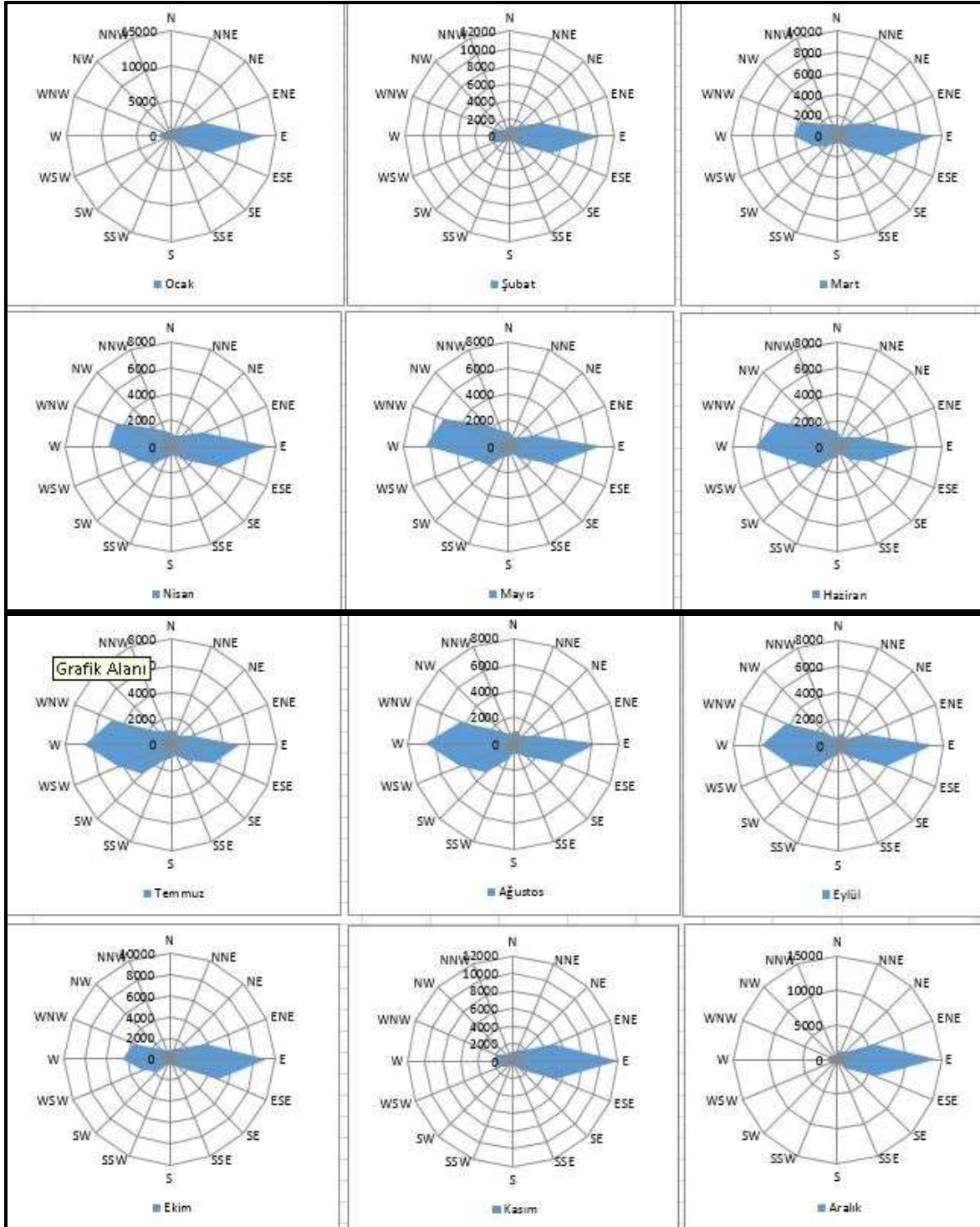
Şekil 31. Aydın Meteoroloji İstasyonuna Ait Esme Sayılarına Göre Aylık Rüzgar Diyagramı
