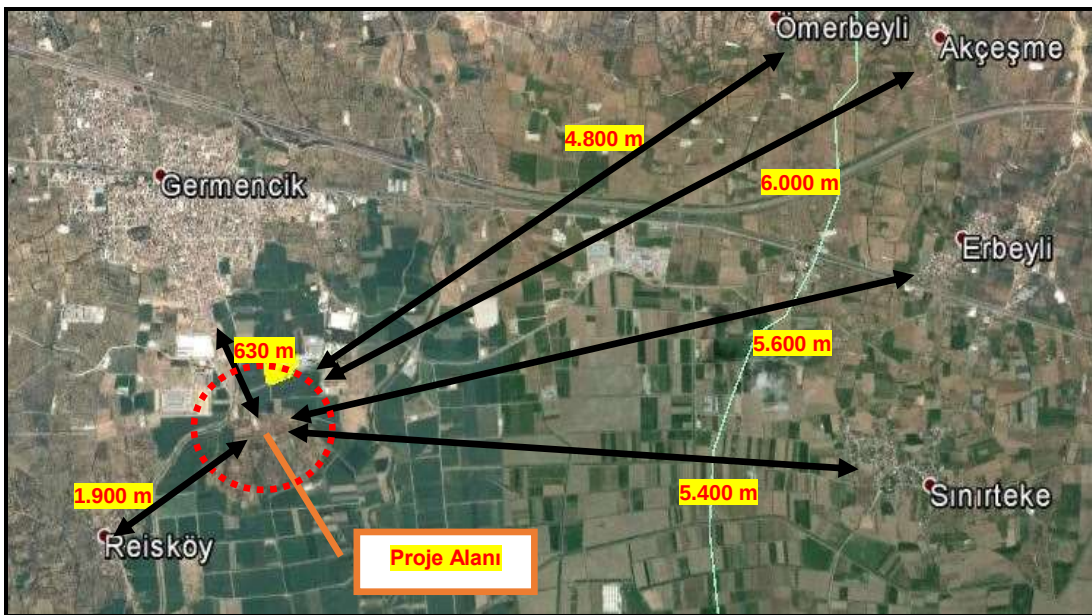
Şekil 16. Proje Alanı ve Proje Alanına En Yakın Yerleşim Yerlerinin Mesafesini Gösterir Uydu Görüntüsü
