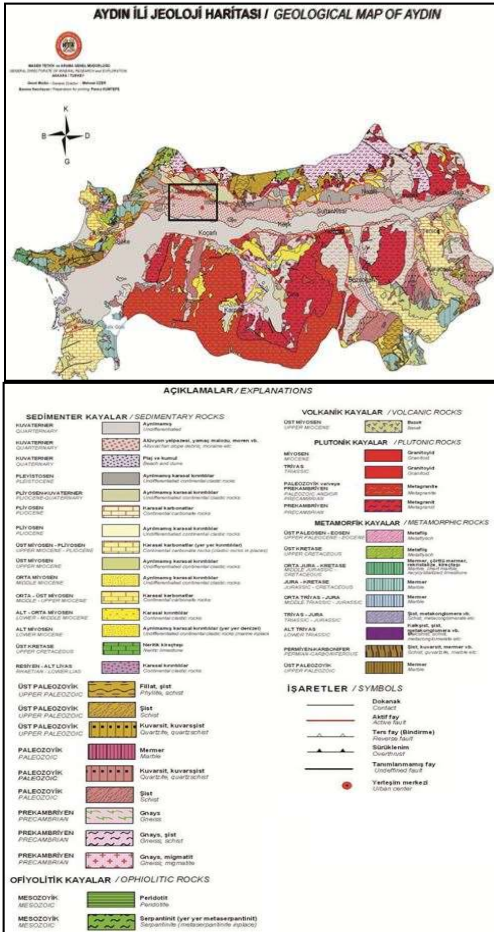
Şekil 33. Aydın İli Jeoloji Haritası
