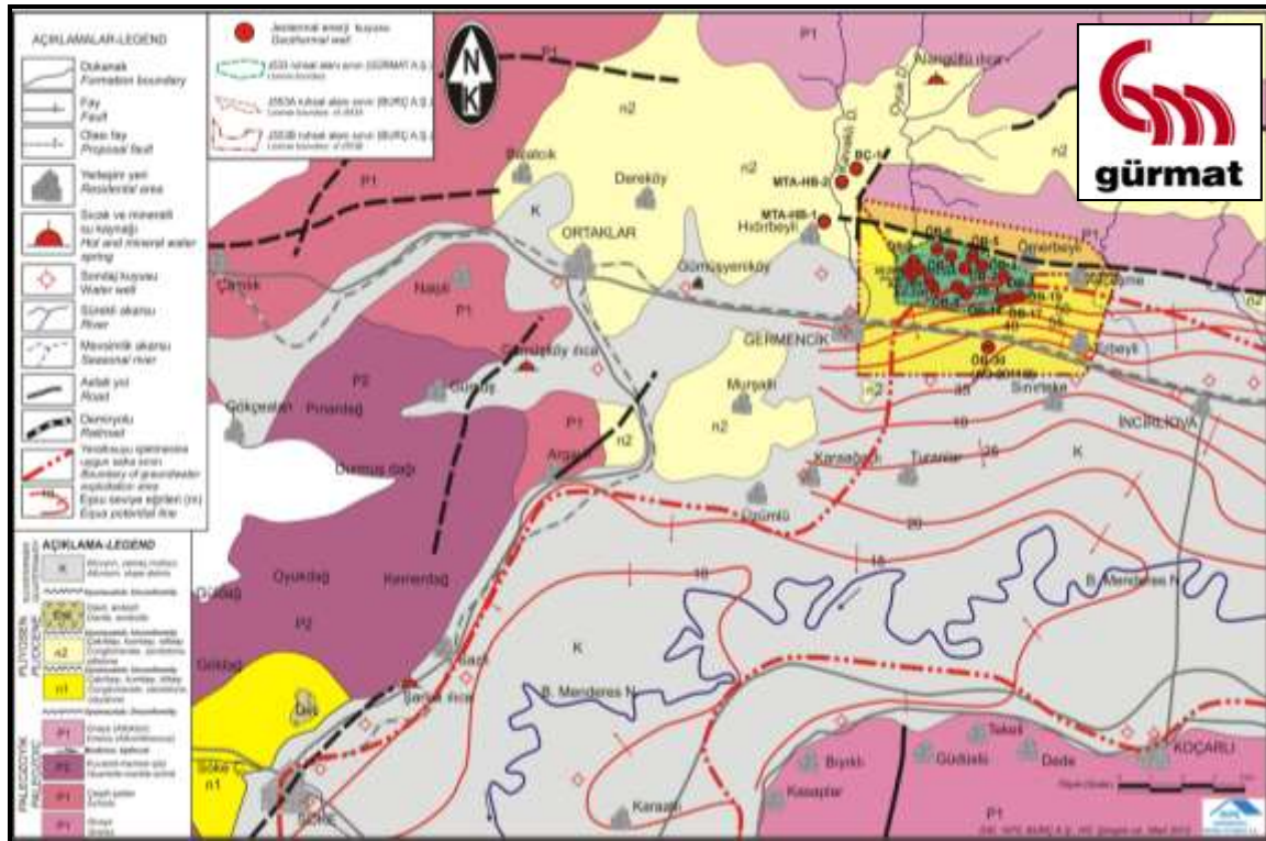
Şekil 48. J-553 Ruhsat Sahasındaki Yeraltı Suları
