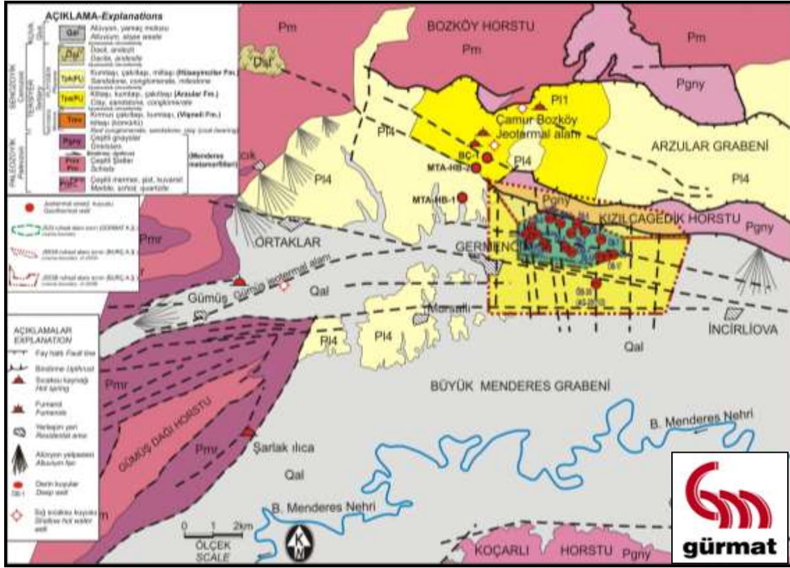
Şekil 36. Proje Alanı ve Yakın Çevresinin Jeoloji Haritası
