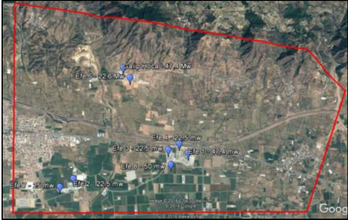
Şekil 106. J-553 Ruhsat Alanında Bulunan Jeotermal Enerji Santralleri
