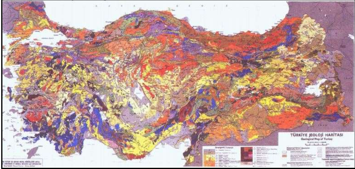
Şekil 32. Türkiye Jeoloji Haritası
