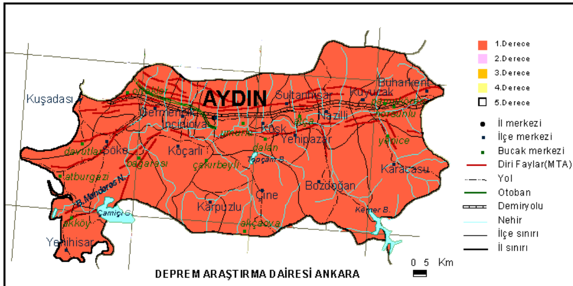
Şekil 41. Aydın Deprem Bölgesi Sınıflandırması
