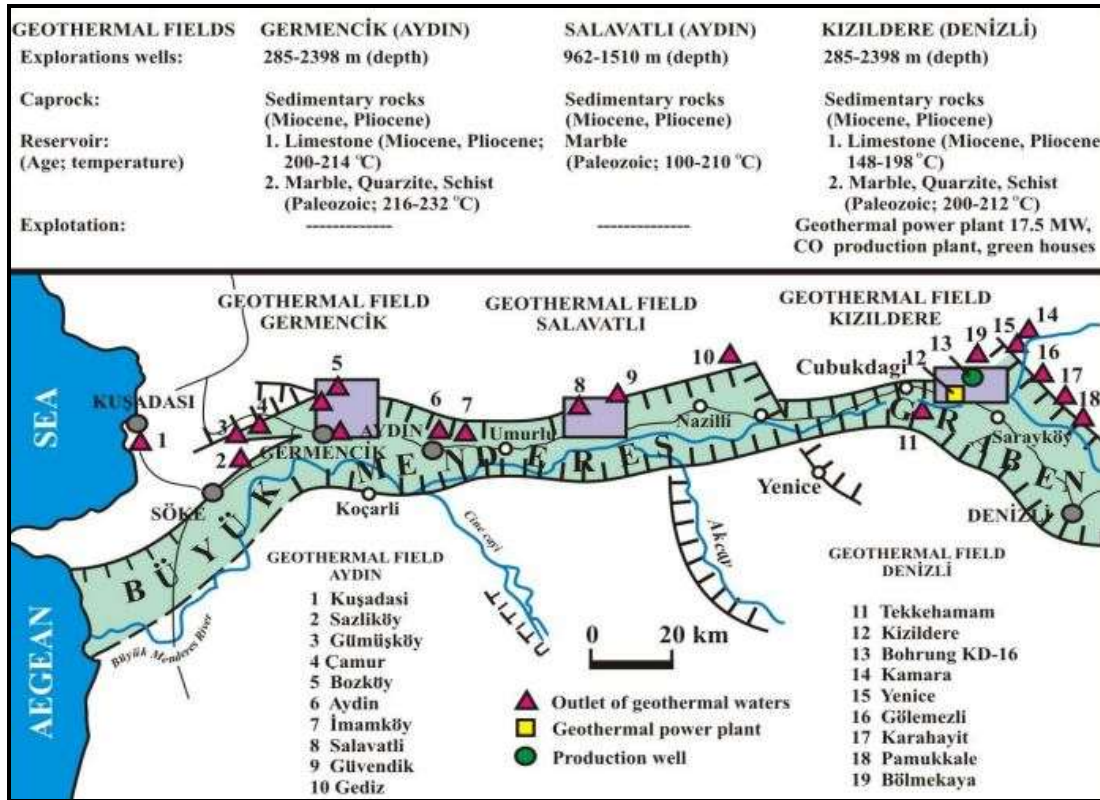
Şekil 35. Büyük Menderes Kıtasal Rift Zonu ve Jeotermal Su Lokasyonları
