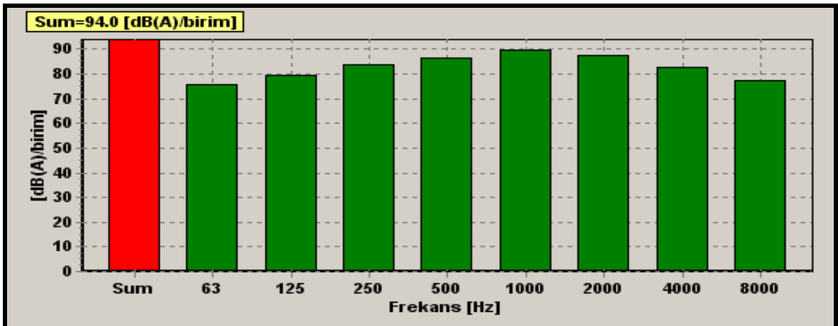
Şekil 99. Kamyona Ait Gürültü Düzeyinin Frekans Analizi
