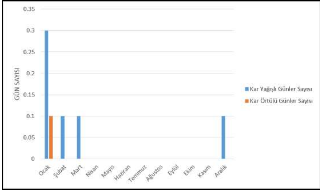
Şekil 21. Aydın Meteoroloji İstasyonuna Ait Kar Yağışlı ve Kar Örtülü Gün Sayıları Grafiği
