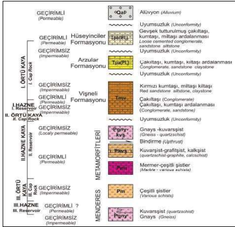
Şekil 45. Germencik Bölgesi Hidrojeolojik Birimleri
