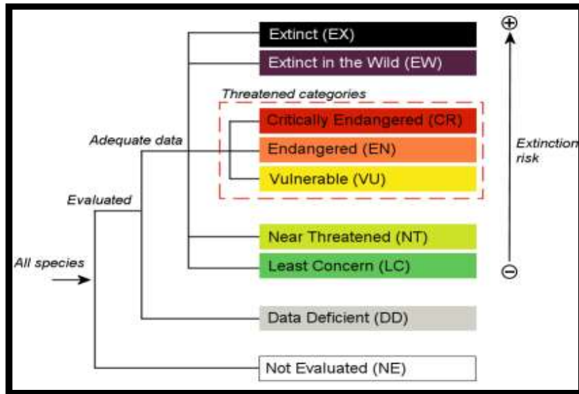
Şekil 74. IUCN Red List Kategorileri Kaynak: www.iucnredlist.org
