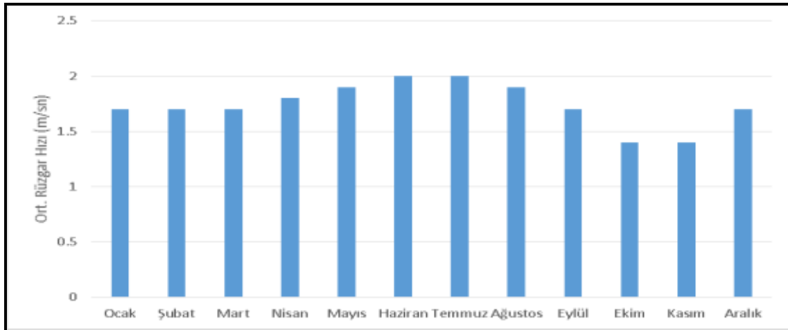
Şekil 25. Aydın Meteoroloji İstasyonu Aylık Ortalama Rüzgar Hızı Grafiği
