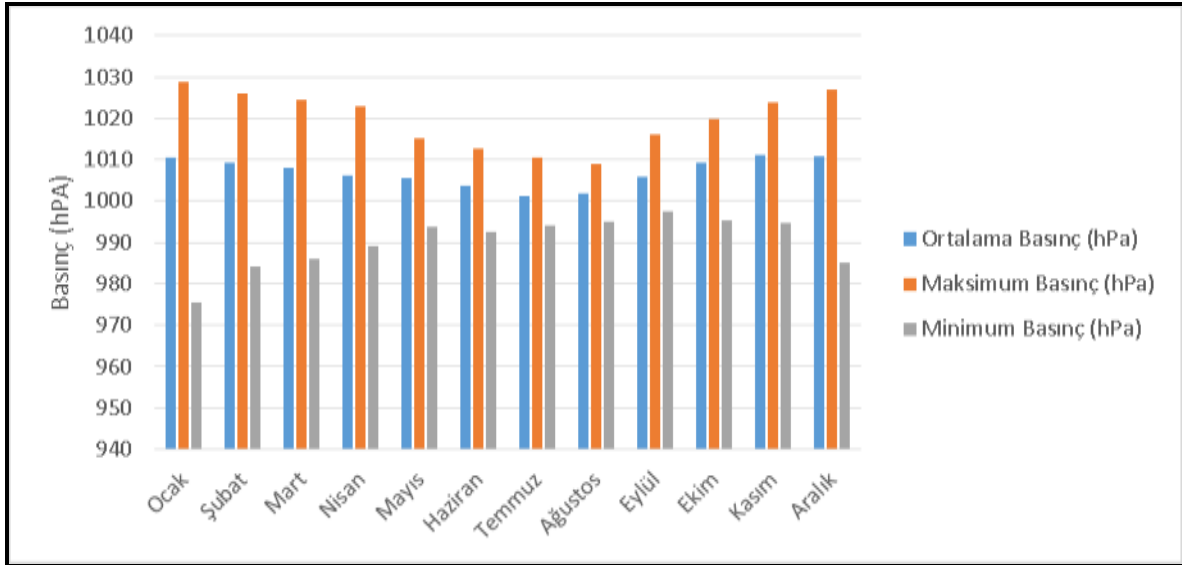
Şekil 17. Aydın Meteoroloji İstasyonuna ait Basınç Değerleri Grafiği
