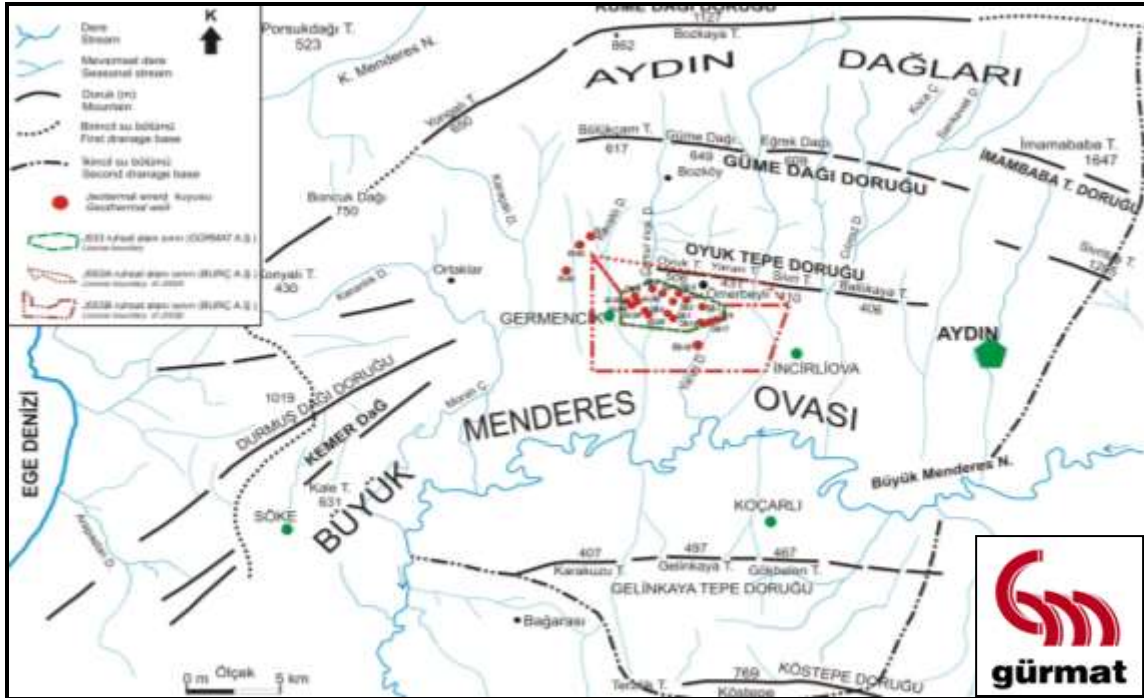
Şekil 46. J-553 Ruhsat Sahasının Hidrografi Haritası
