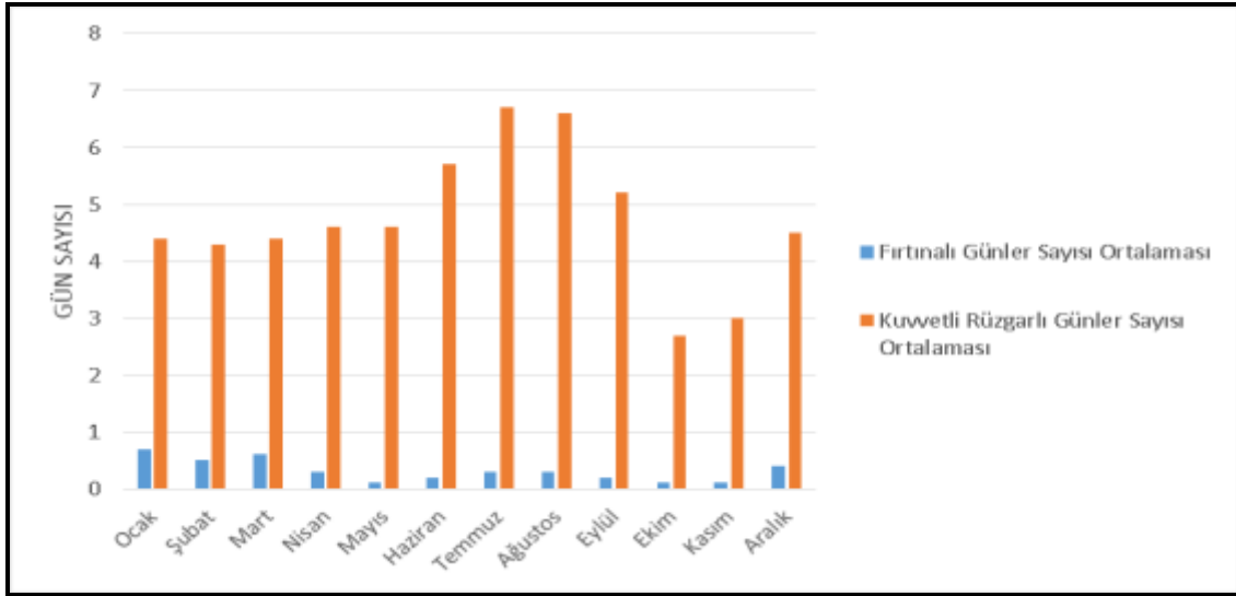
Şekil 27. Aydın Meteoroloji İstasyonuna ait Fırtınalı ve Kuvvetli Rüzgarlı Günler Grafiği
