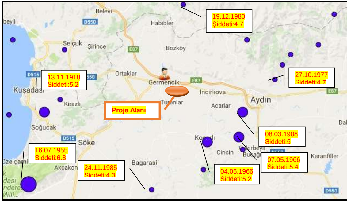
Şekil 44. Proje Alanının Yer Aldığı Bölgedeki Büyük Depremlerin Tarih ve Şiddetleri
