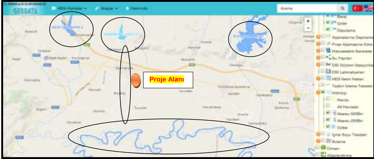
Şekil 72. Proje Alanı ve Yakın Çevresinde Yer Alan Baraj, Göl, Gölet, Akarsuları Gösterir Harita
