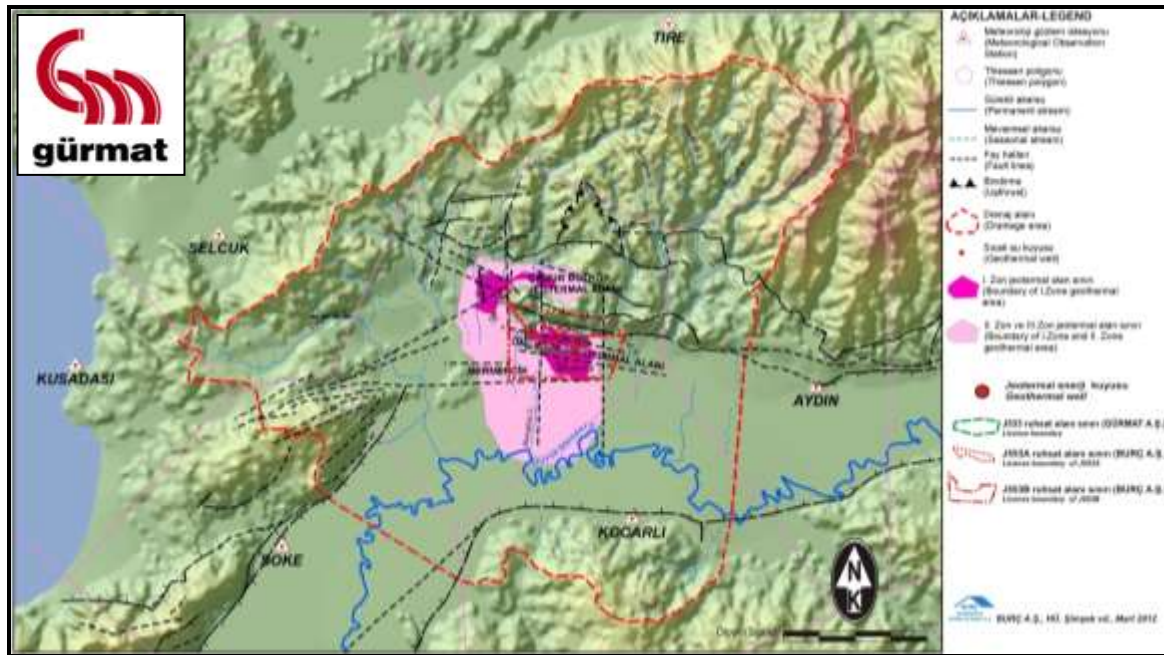
Şekil 49. J-553 Ruhsat Sahasının Beslenme Alanı
