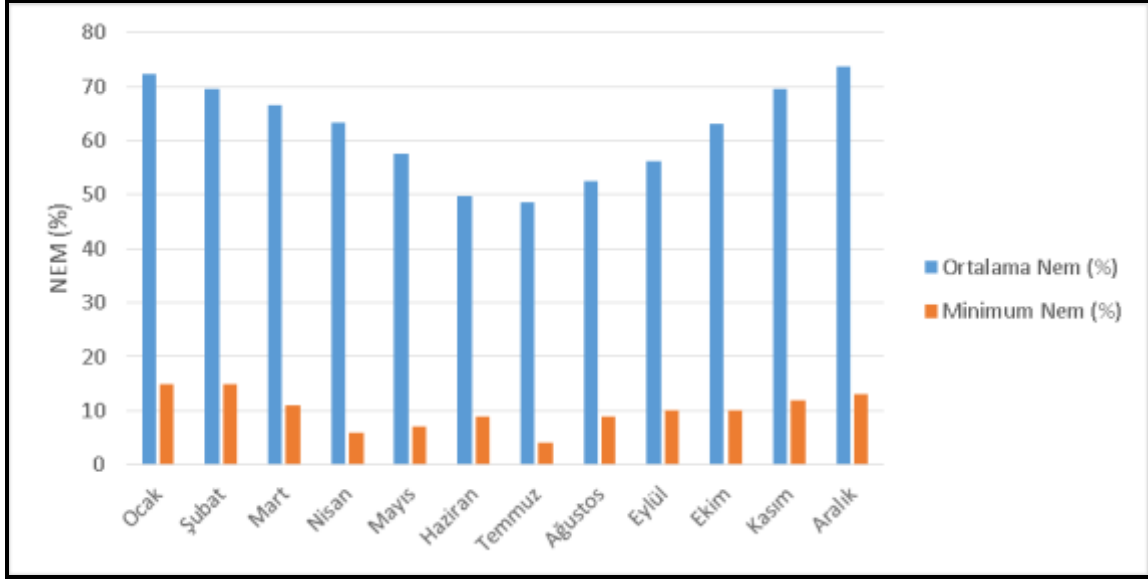
Şekil 20. Aydın Meteoroloji İstasyonuna Ait En Düşük ve Ortalama Nem Verilerinin Grafiksel Gösterimi
