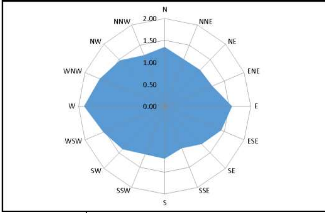
Şekil 29. Aydın Meteoroloji İstasyonuna Ait Ortalama Rüzgar Hızına Göre Yıllık Rüzgar Diyagramı
