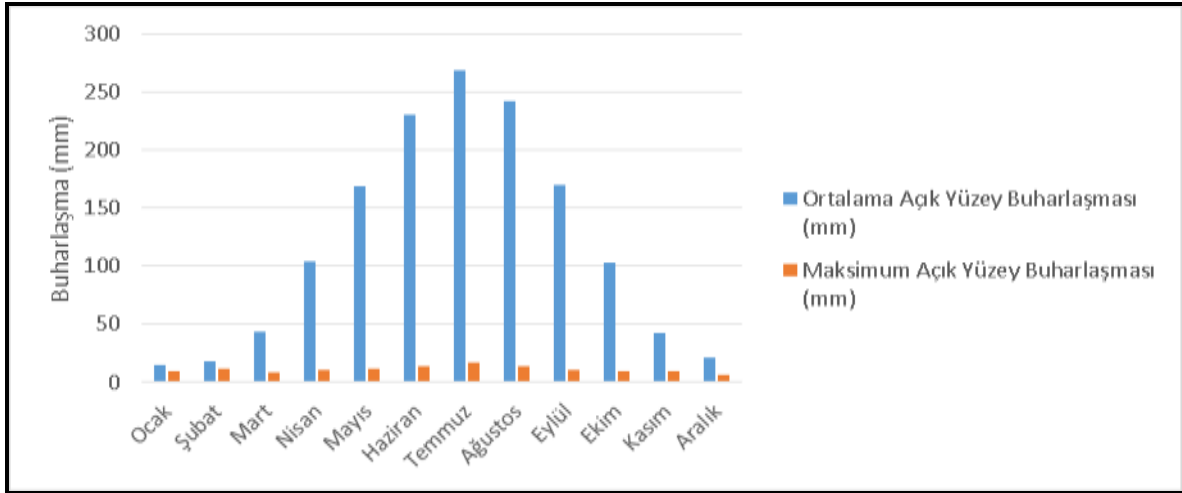
Şekil 24. Aydın Meteoroloji İstasyonu Ortalama ve Maksimum Açık Yüzey Buharlaşması Verilerinin Grafiksel Gösterimi
