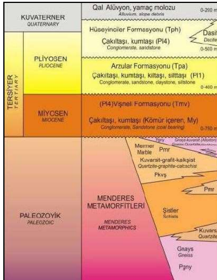
Şekil 34. Proje Alanı ve Çevresi Genelleştirilmiş Stratigrafik Sütun Kesiti
