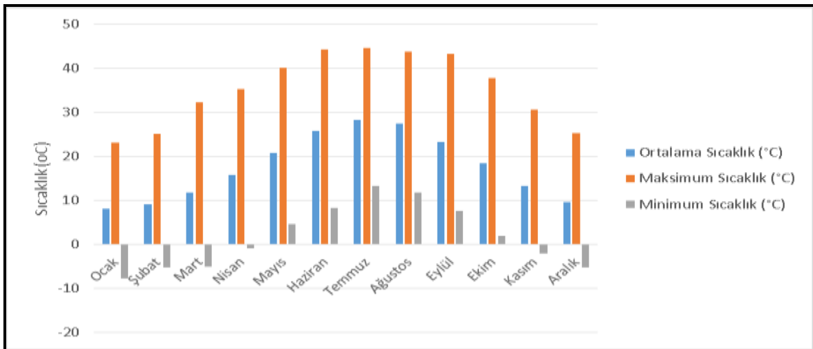
Şekil 18. Aydın Meteoroloji İstasyonundan Elde Edilen Aylık Sıcaklık Dağılımları Grafiği
