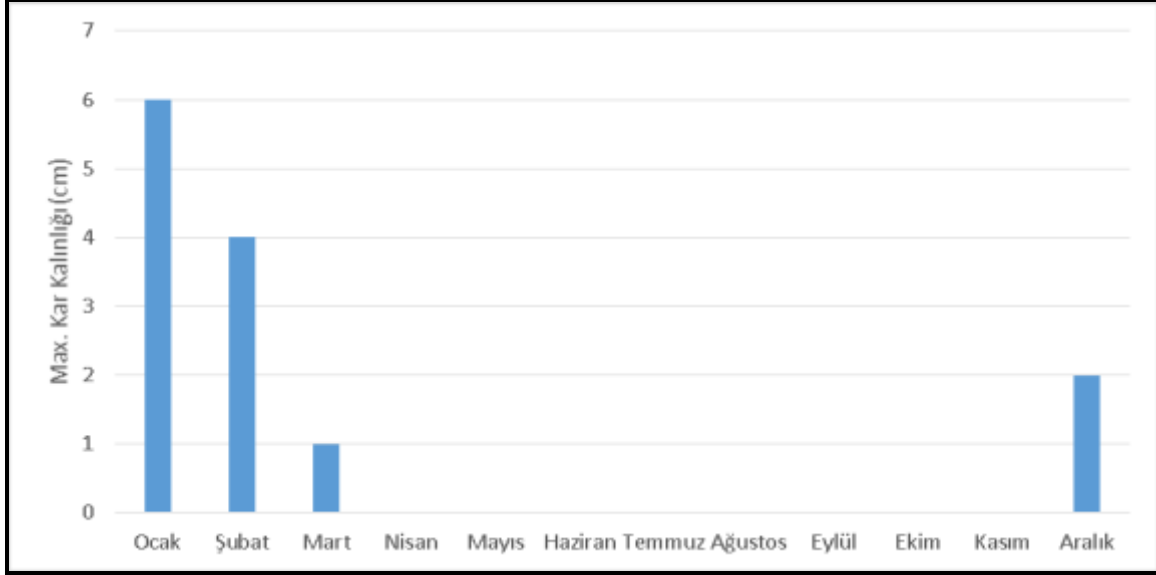
Şekil 23. Aydın Meteoroloji İstasyonuna Ait Maksimum Kar Kalınlığı Aylara Göre Dağılım Grafiği
