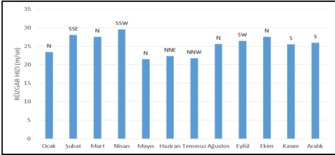
Şekil 26. Aydın Meteoroloji İstasyonu Maksimum Rüzgar Hızı Grafiği
